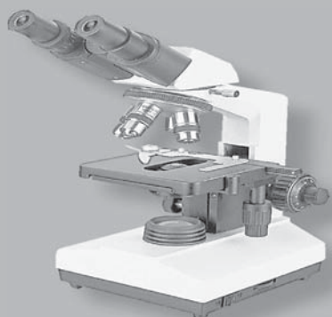
显微镜
