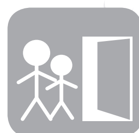
设定逃生路线
