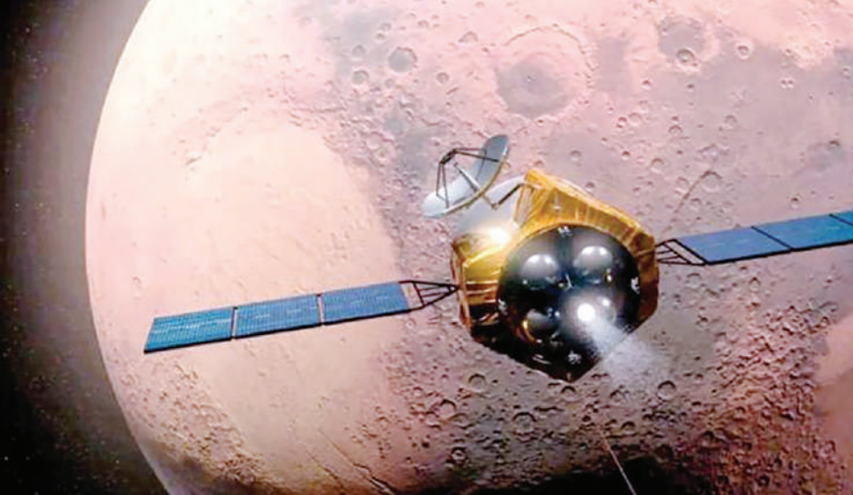
天问一号：惊鸿一瞥观测到阿特拉斯。
