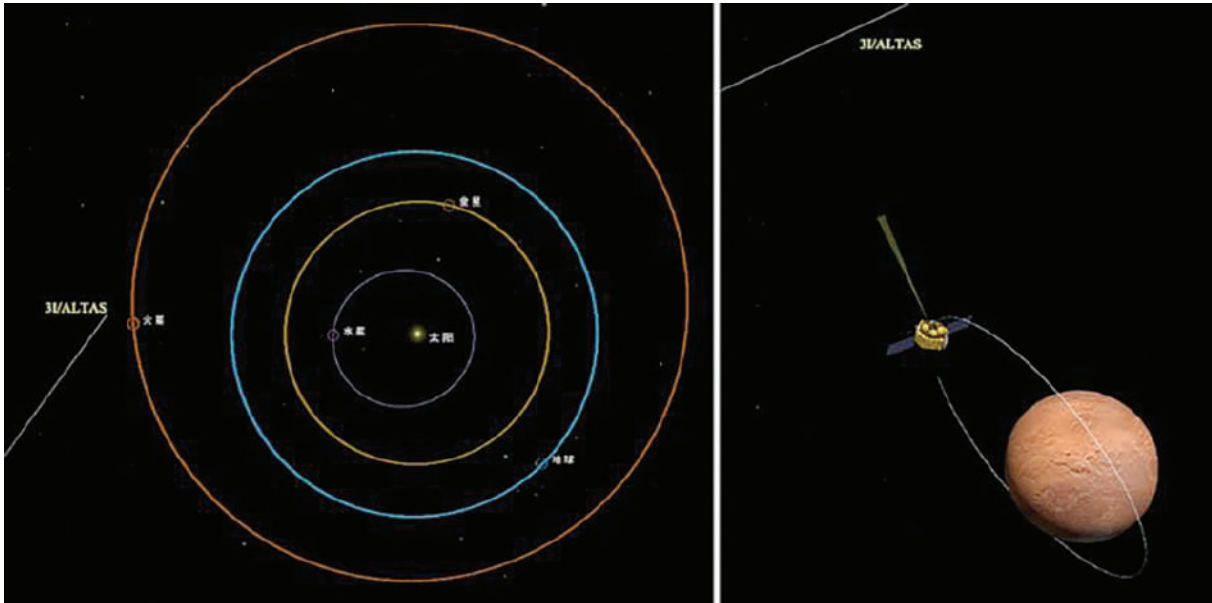
阿特拉斯进入太阳系示意图：联合观测。
