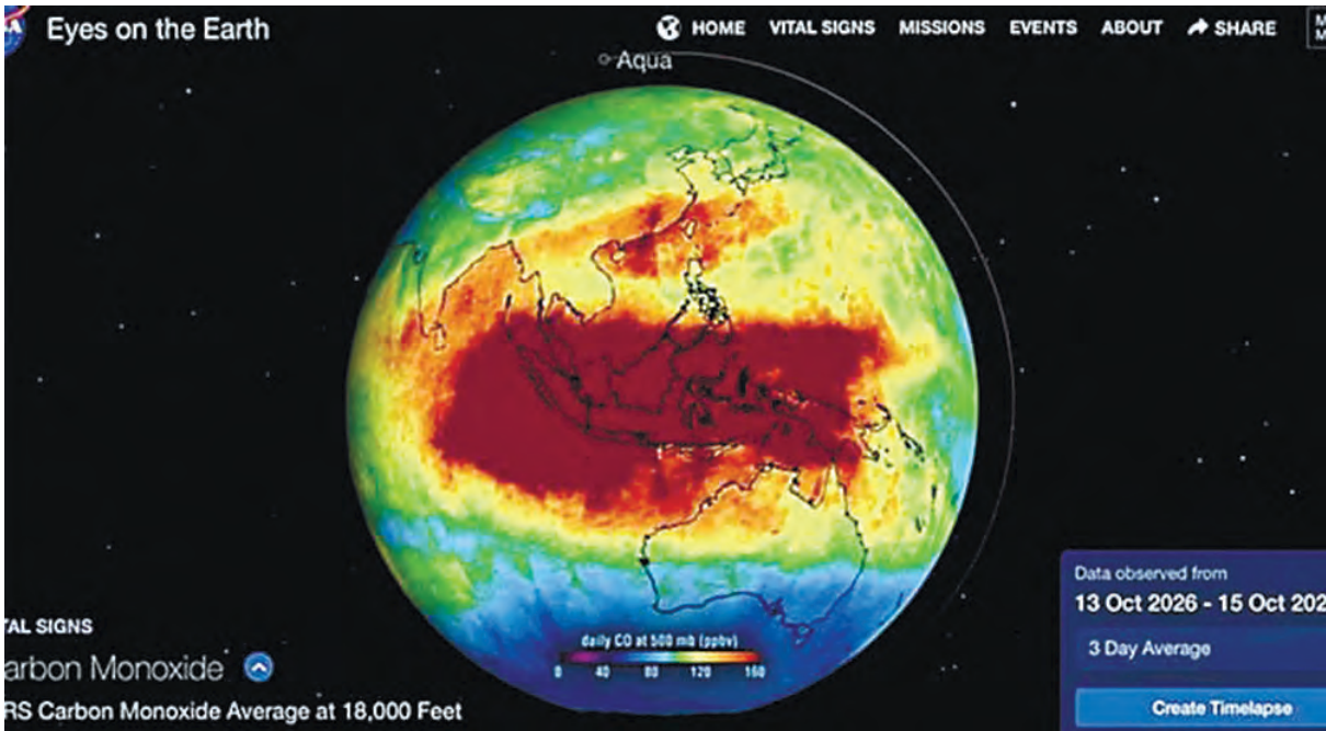
NASA卫星分析图：印尼、大马一带空气污染严重。
